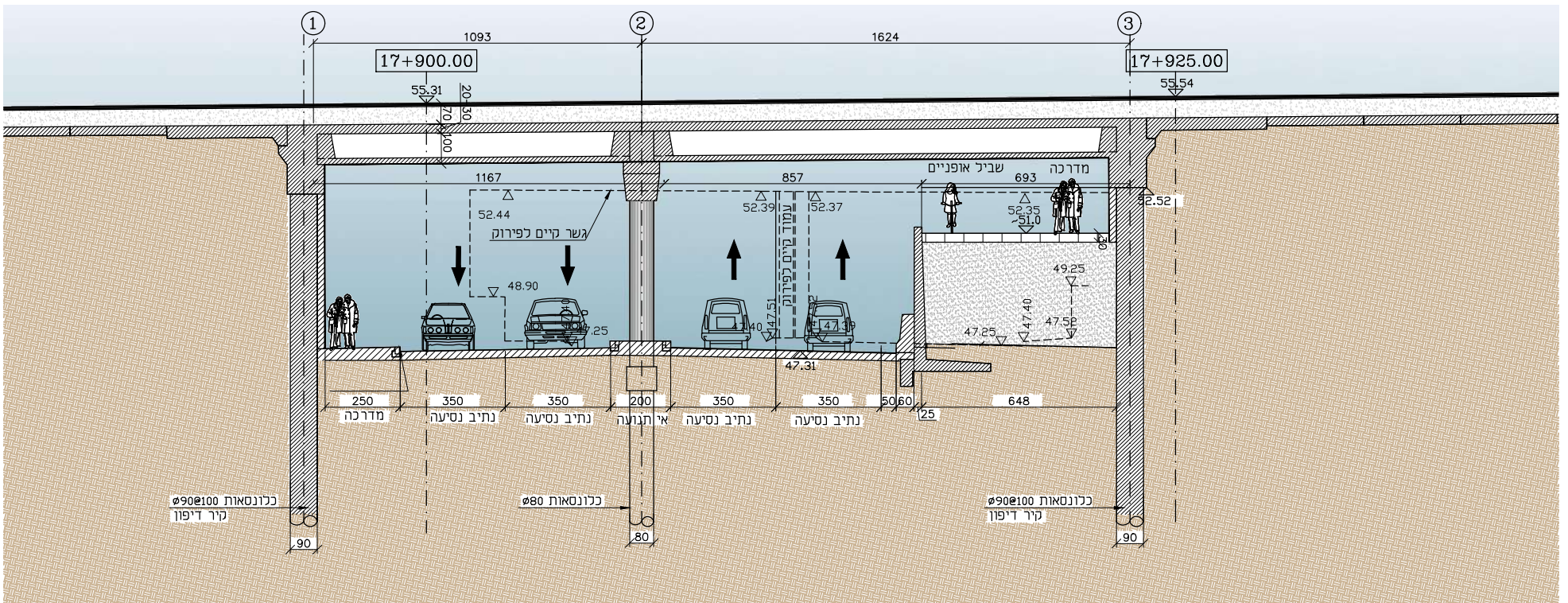
חתך 3-3 לרוחב המעבר המשוקע, לרוחב הגשר 1:200
