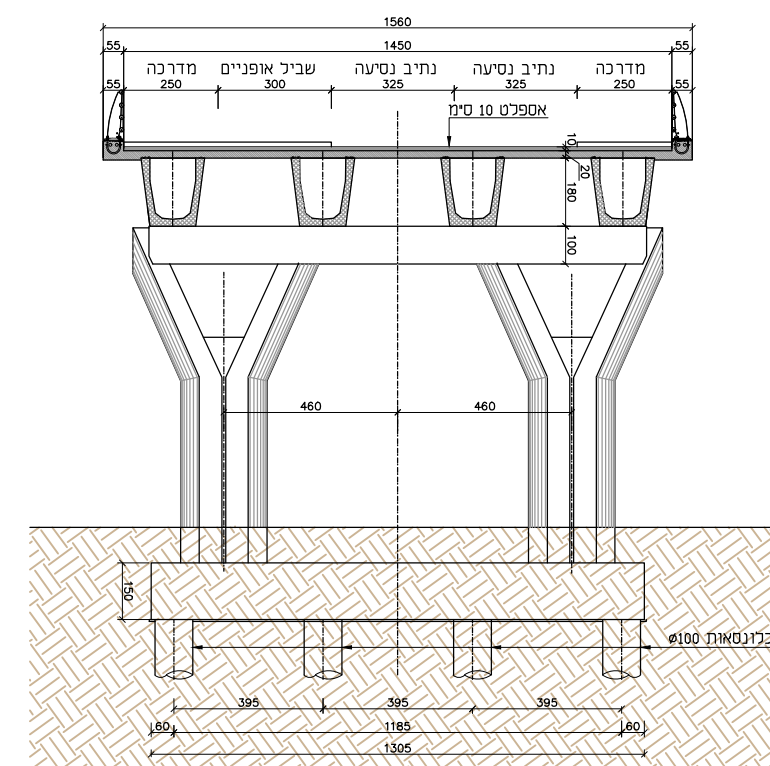
חתך בנציבים 2 3
