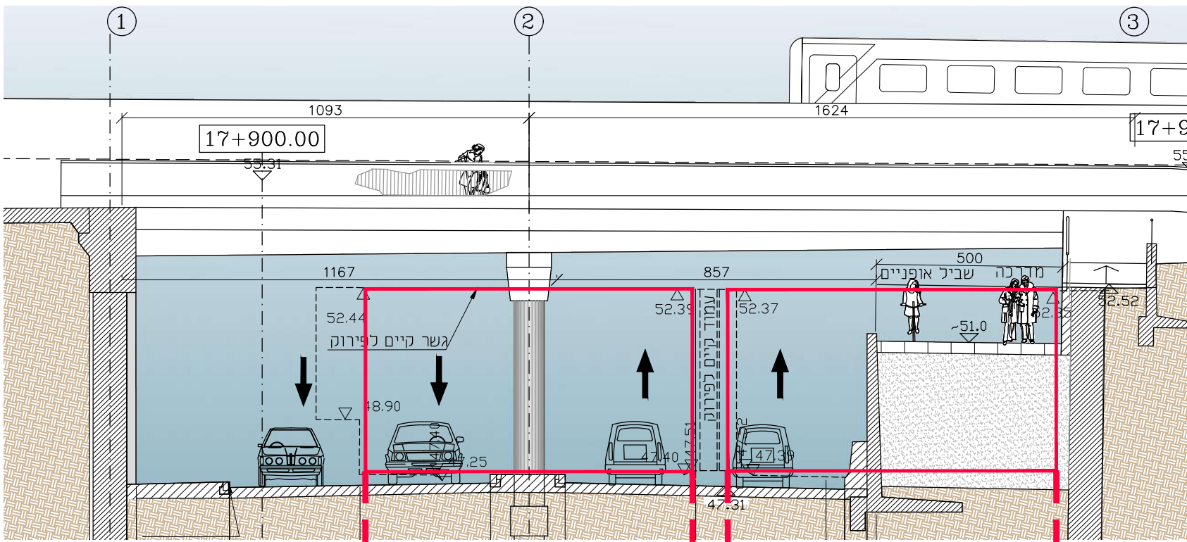
חתך בגשר מתוכנן על רקע קיים
