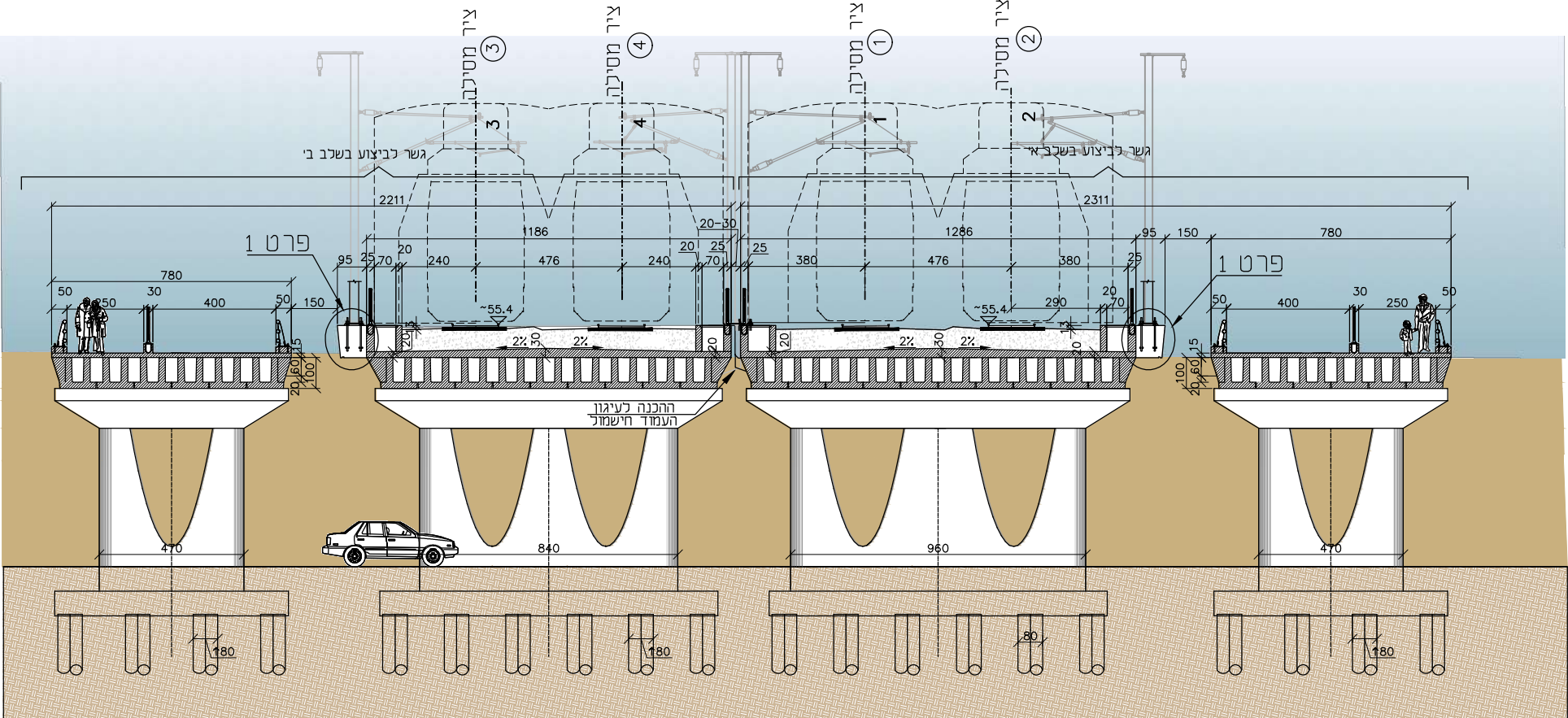
חתך 1-1 לרוחב דרך נציב אמצעי 1:200
