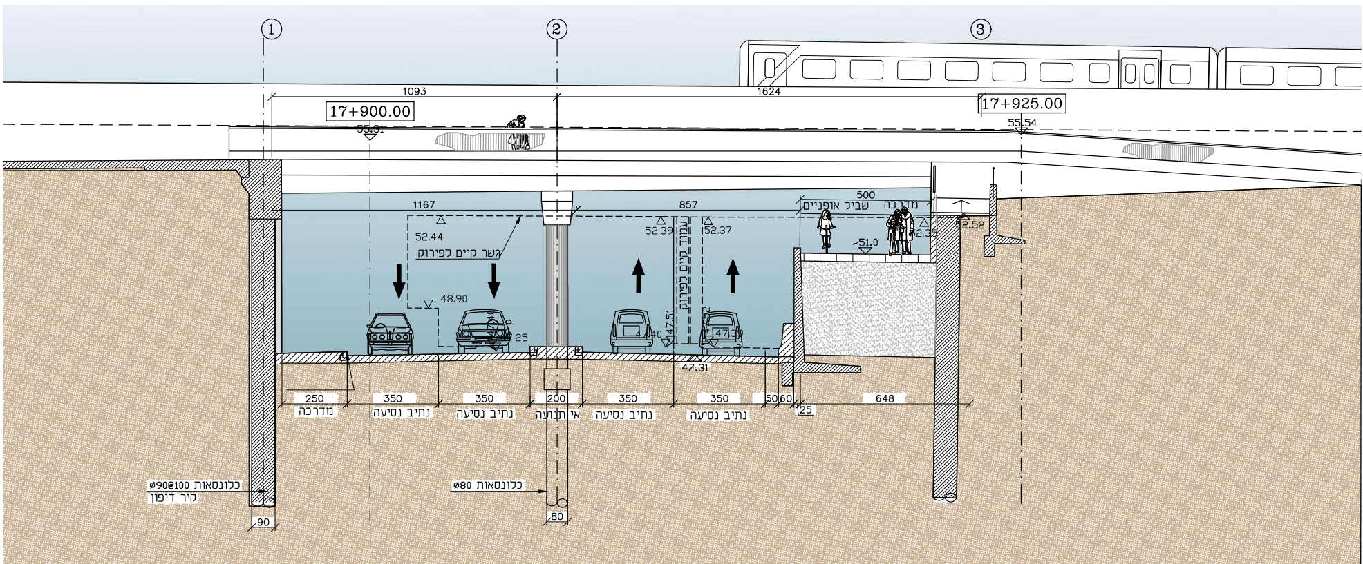
חתך 2-2 לרוחב המעבר המשוקע, לפני הגשר 1:200
